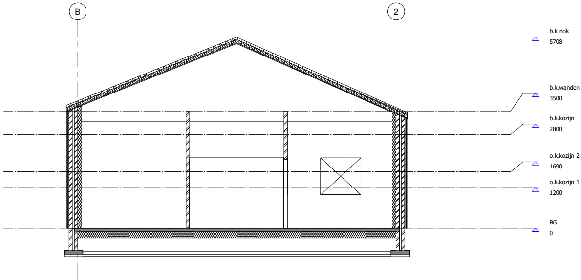
6 Doorsnede 1 : 50
