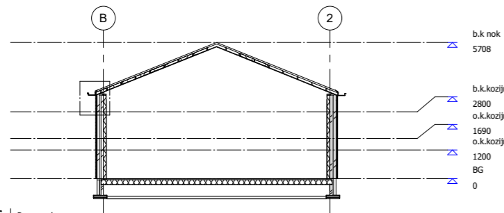
6 Doorsnede 1 : 100
