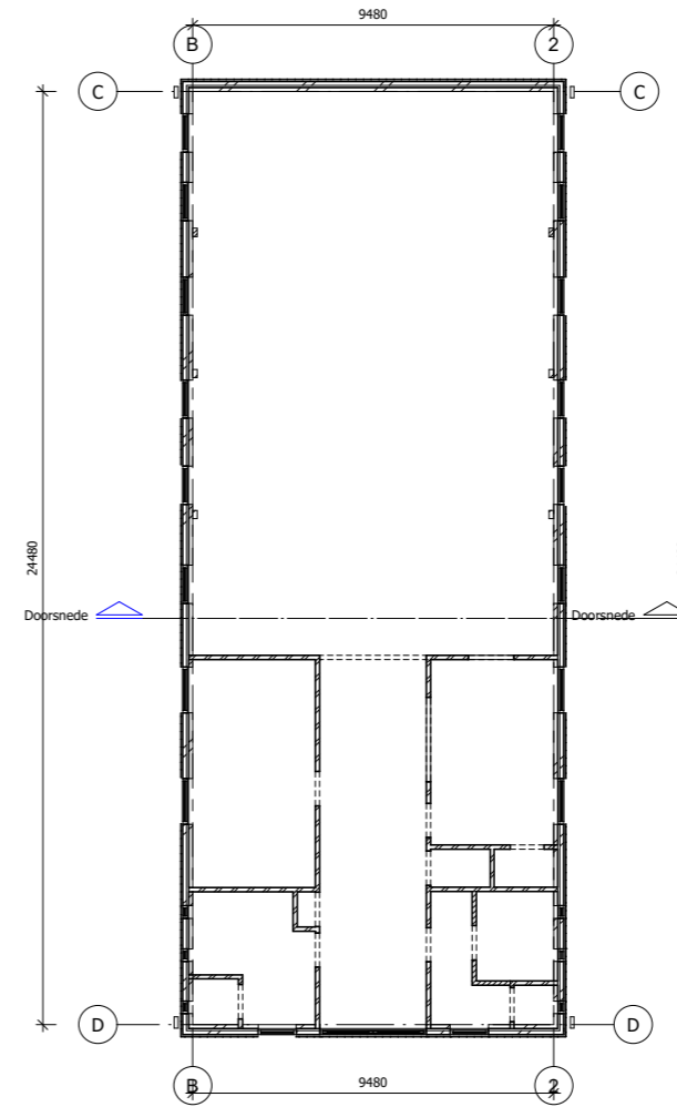
7 plattegrond 1 : 100
