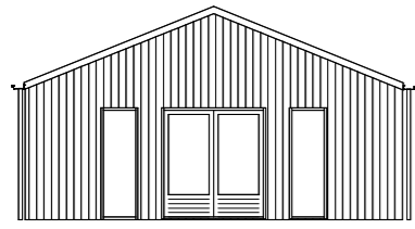
4 Vooraanzicht 1 : 100
