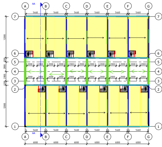
Eerste verdieping
