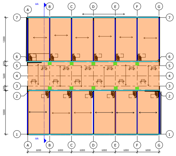
Begane grondvloer
